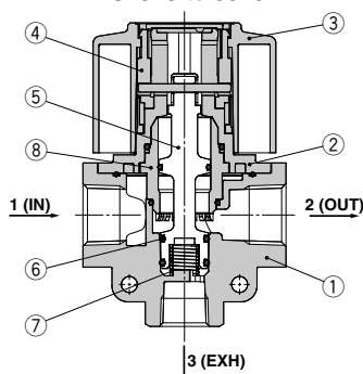
VHS2510 to 5510-A
